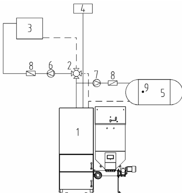
Obr. č. 9 Blokové schéma instalace ÚT v soustavě se čtyřcestným ventilem a čerpadlem TUV
