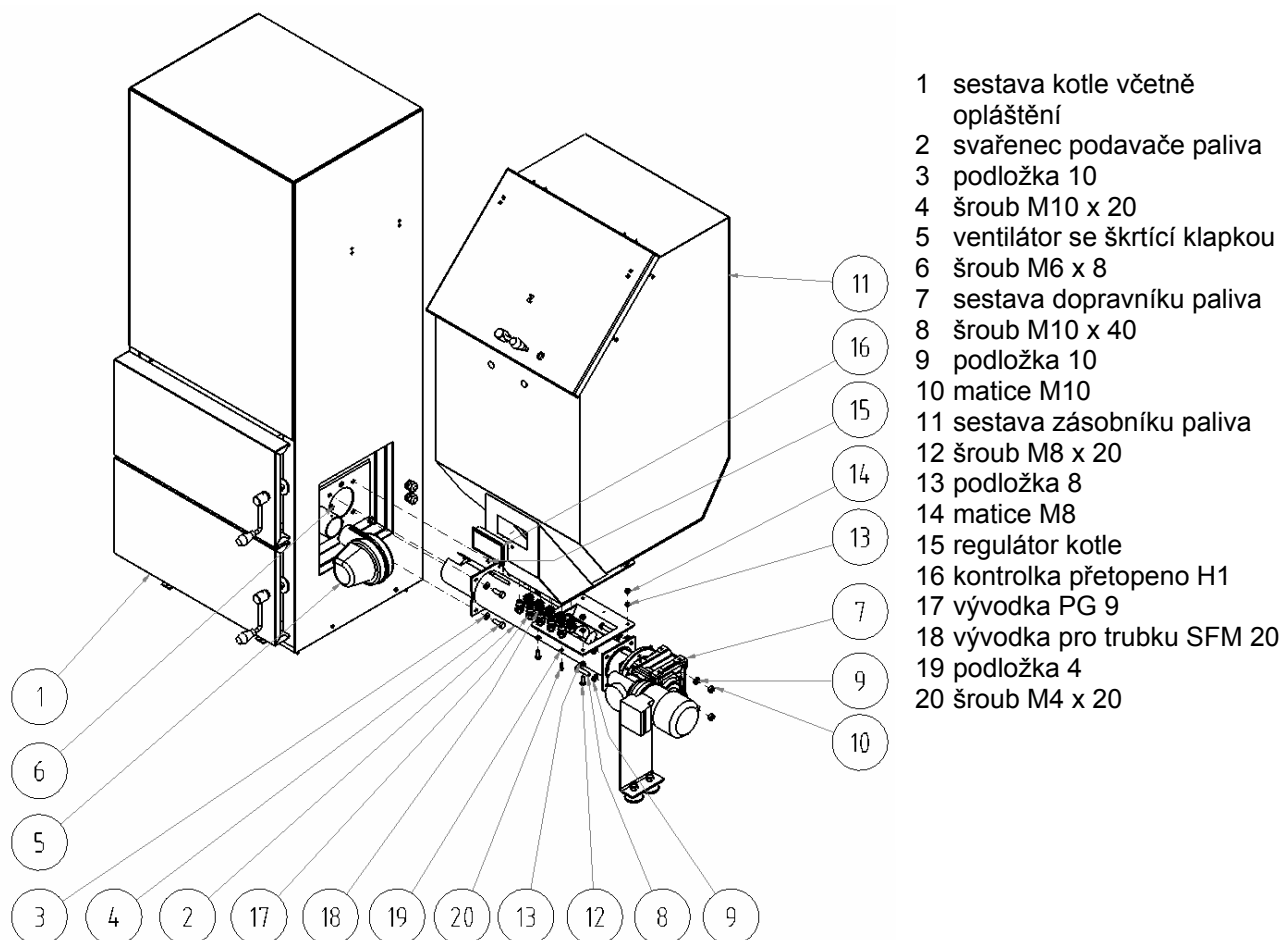
Obr. č. 7 Montáž zásobníku a podavače
