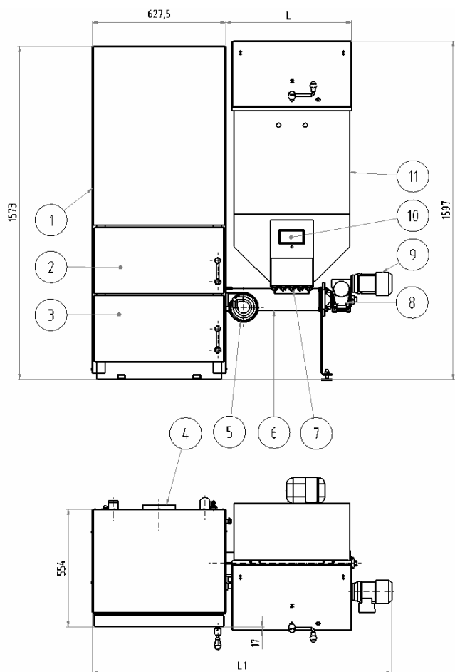
Obr. č. 1 Schéma kotle VIADRUS EKORET (pravé provedení)
