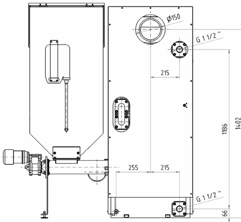
Obr. č. 8 Připojovací rozměry kotle VIADRUS EKORET
