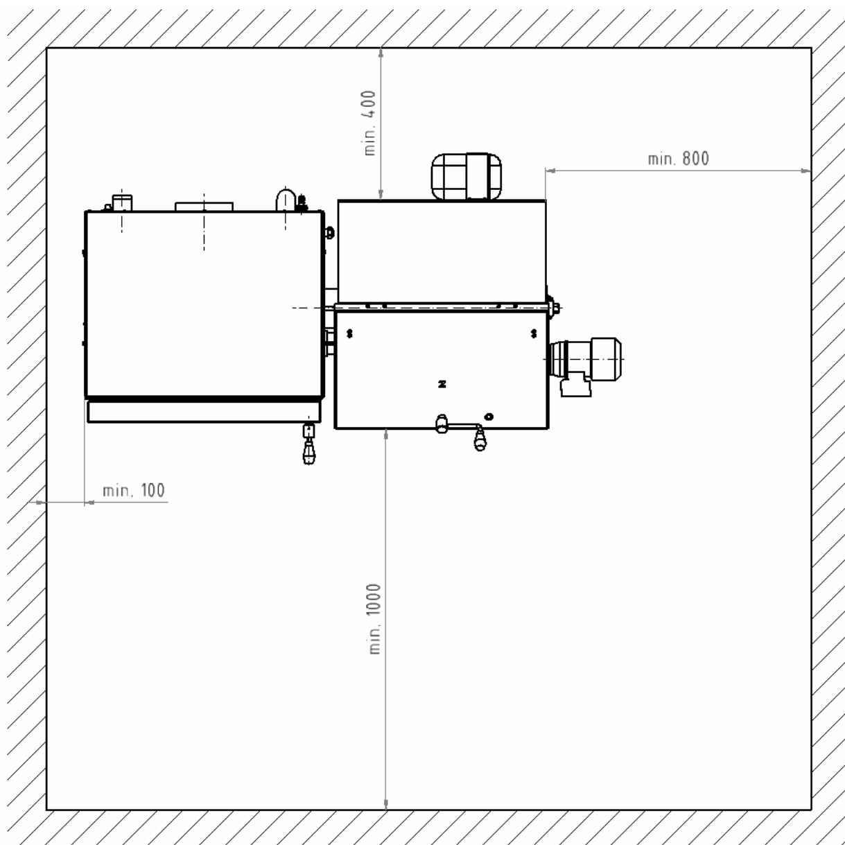
Obr. č. 3 Umístění kotle VIADRUS EKORET v kotelně
