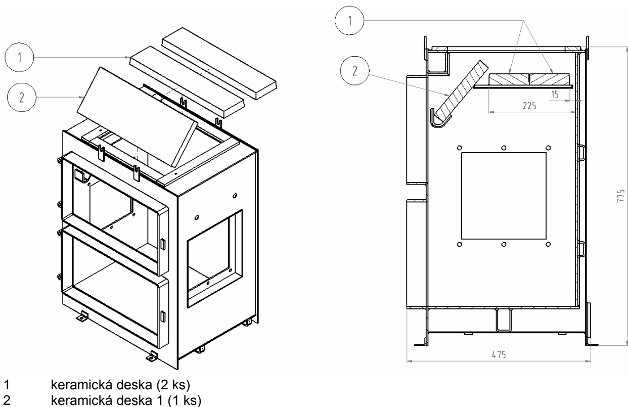
Obr. č. 5 Řez hořákovým prostorem kotle 15 a 25 kW
