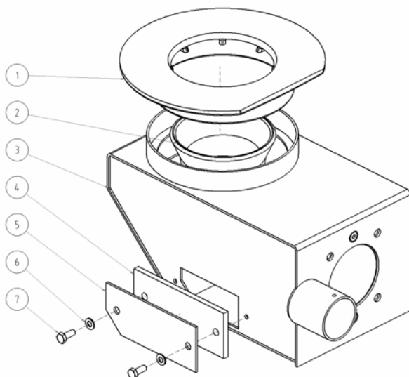
Obr. č. 2 Hořák se směšovačem
