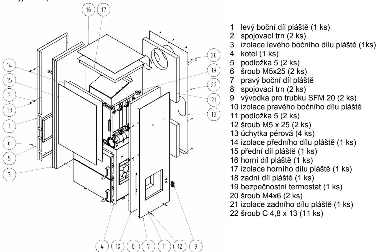
Obr. č. 6 Montáž opláštění VIADRUS EKORET
